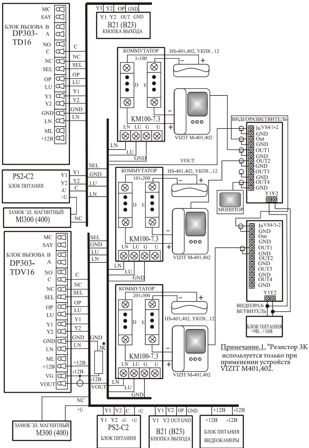
Рис.3 Пример схемы подключения DP303-TDV16 в составе домофонного комплекса.
