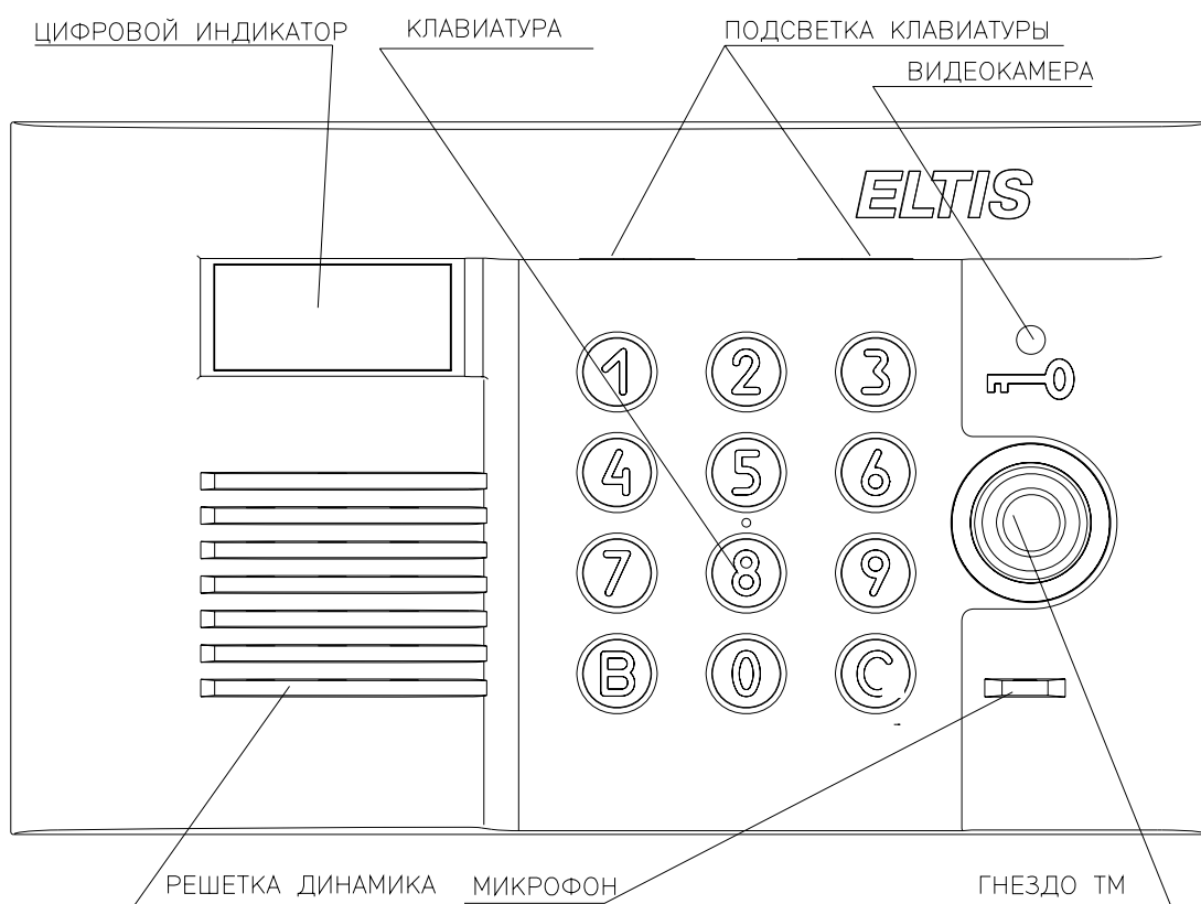
Рис.1 Внешний вид со стороны лицевой панели блока вызова DP303-TDV16.
