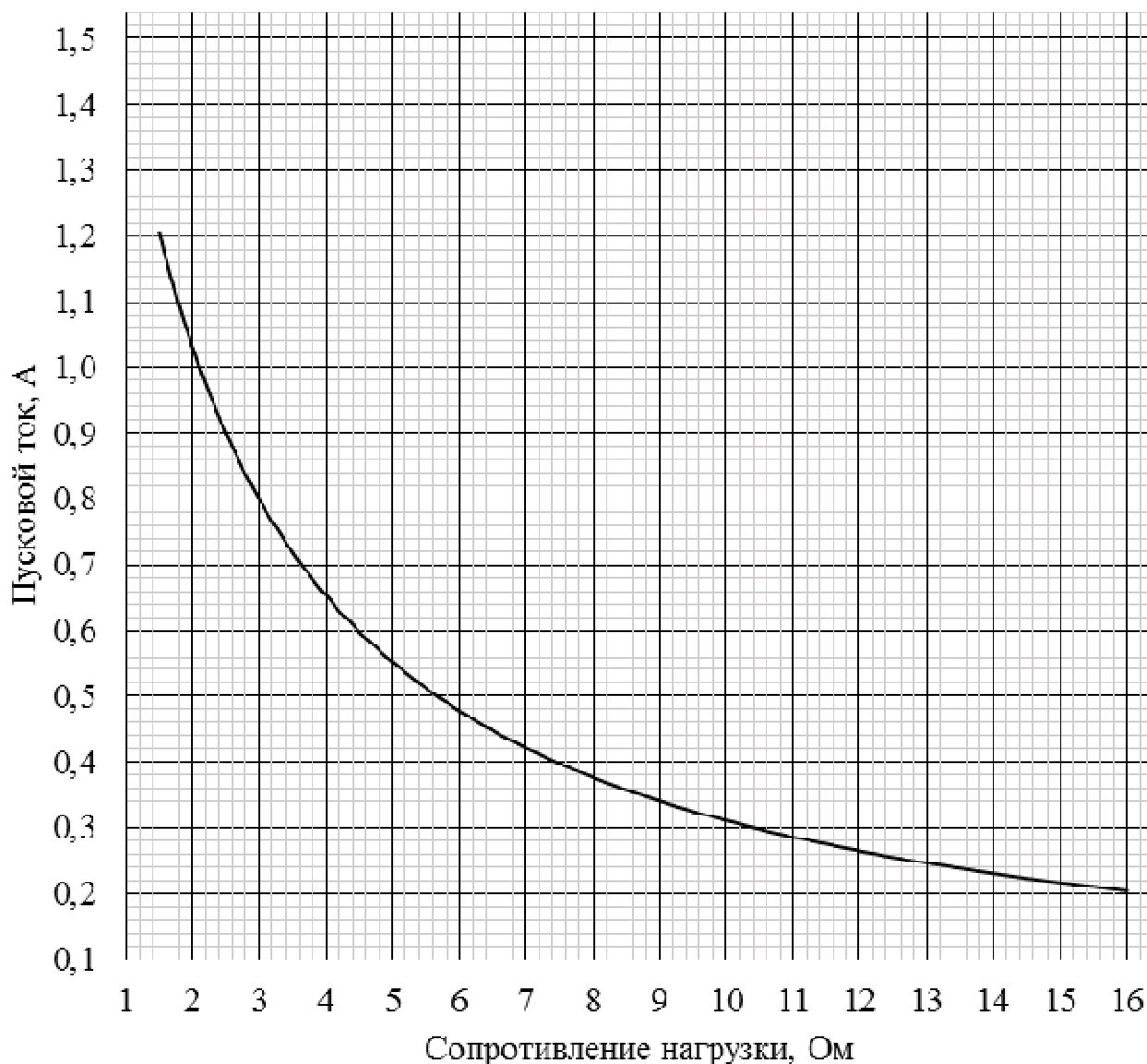
Рисунок 1 – График зависимости пускового тока от сопротивления нагрузки
