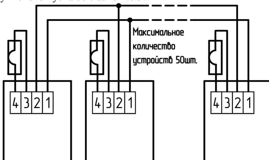
Рисунок 4 – Схема группового включения устройств
