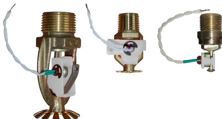
Установка УПП «Старт-1» на оросителе
