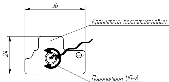
Внешний вид и габаритные размеры УПП «Старт-1» (исполнения 1 и 2)
