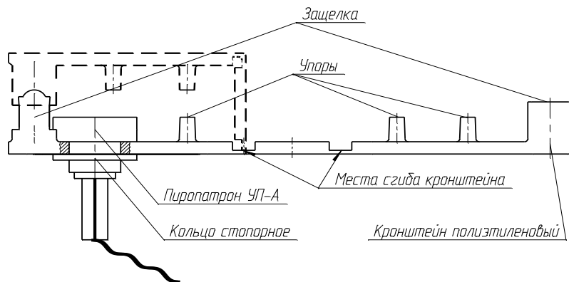
Установка УПП «Старт-1» на оросителе
